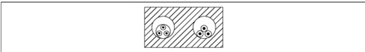
Figuur 2.11. Plaatsingswijze «holle blok»
