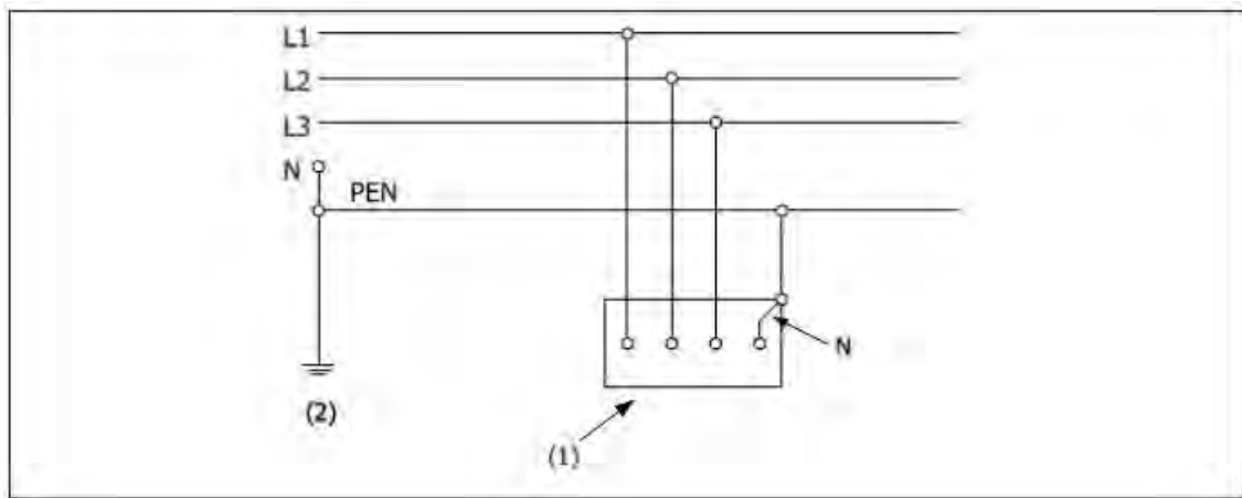
Figuur 2.2. TN-C-systeem
