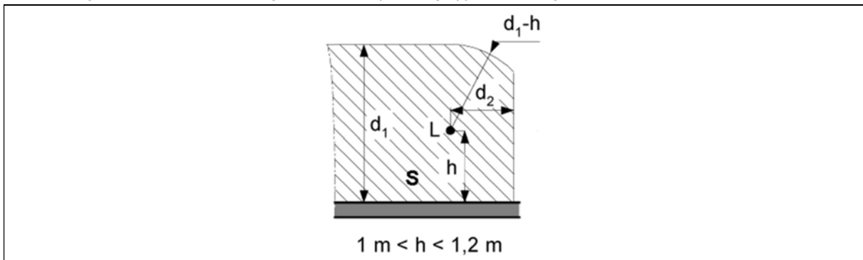
Figuur 2.7. Genaakbaarheidsgebarit: het verplaatsingsoppervlak is begrensd door een materieel element
