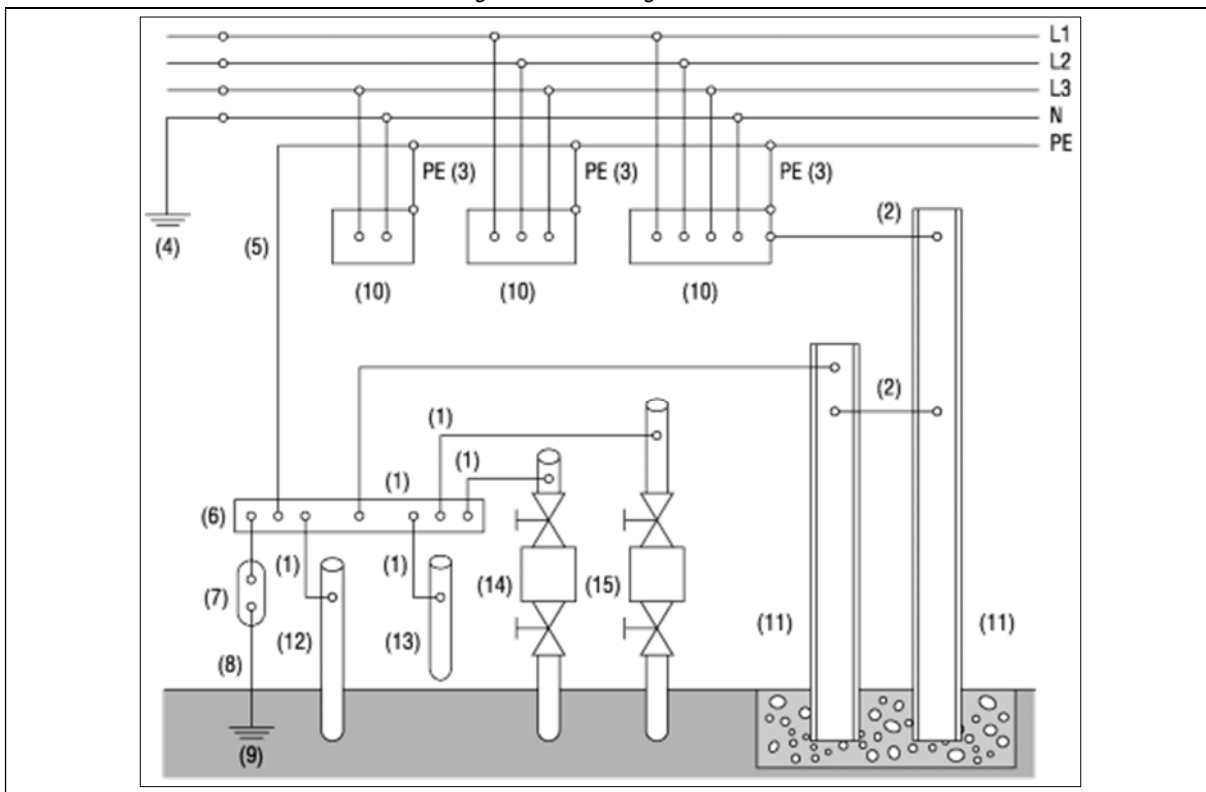
Figuur 2.10. Aardingsinstallatie
