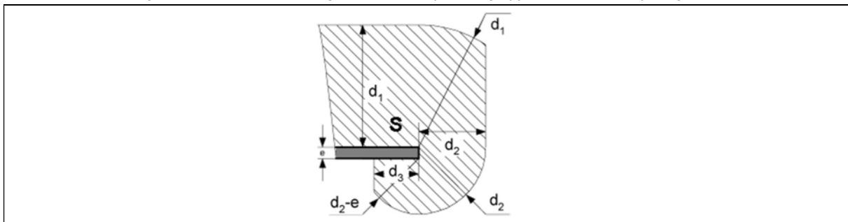
Figuur 2.7. Genaakbaarheidsgebarit: het verplaatsingsoppervlak is begrensd door een materieel element
