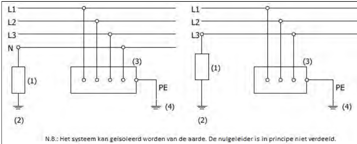
Figuur 2.5. IT-systeem
