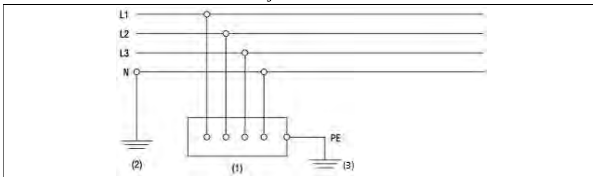
Figuur 3.4. TT-net
