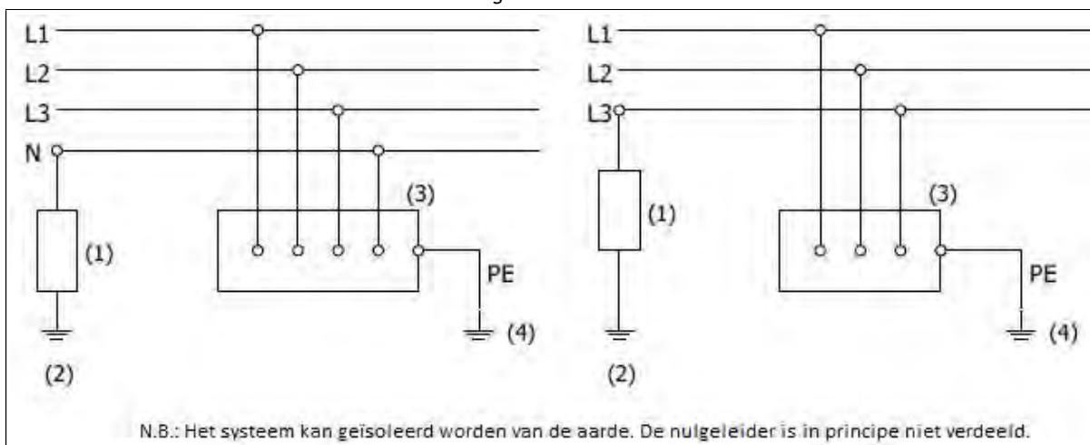
Figuur 3.5. IT-net
